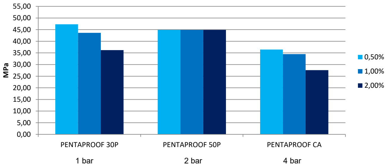
Preservazione delle RCK a 28 giorni (Uni EN 1015-11)
