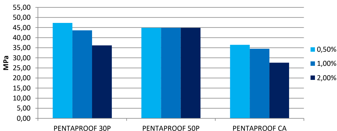
Préservations des RCK à 28 jours (Uni EN 1015-11)
