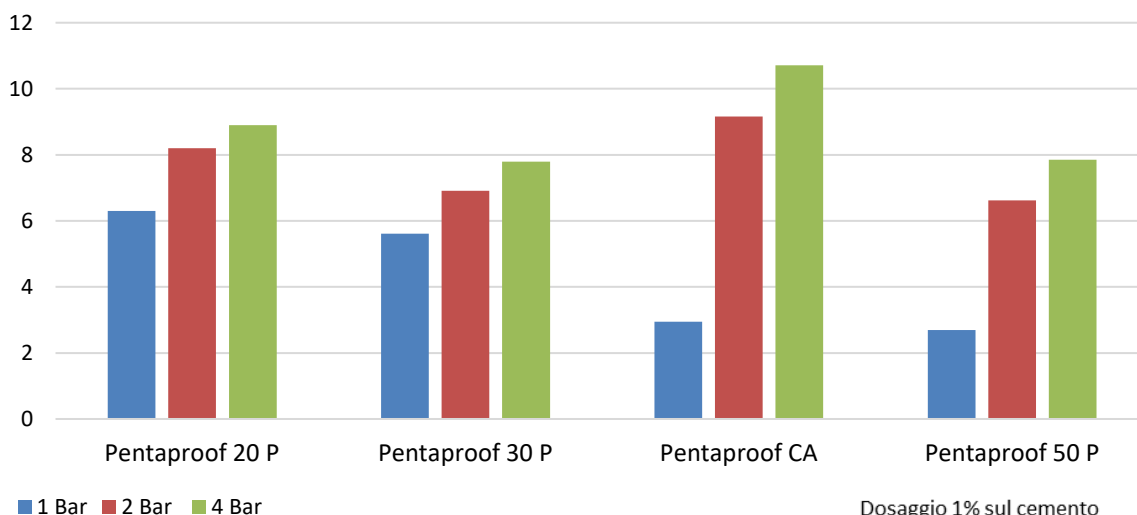
Assorbimento d'acqua dei vari prodotti Pentaproof al variare della pressione dell'acqua (dosaggio 1,0% sul cemento)
