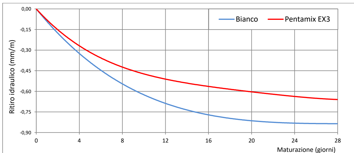
Azione del Pentamix EX sui ritiri idraulici in una malta standard Pentachem
